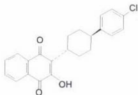
Atovaquone
